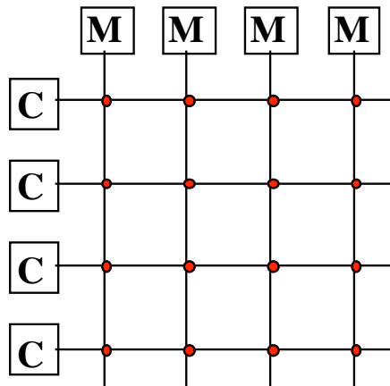
Kreuzschienenverteiler
